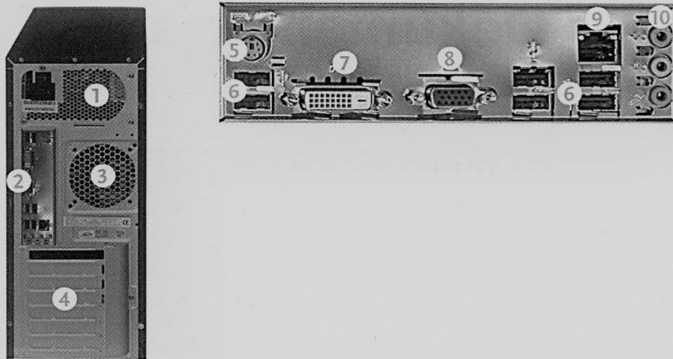
Rys. 98.2. Jednostka centralna (tył)
