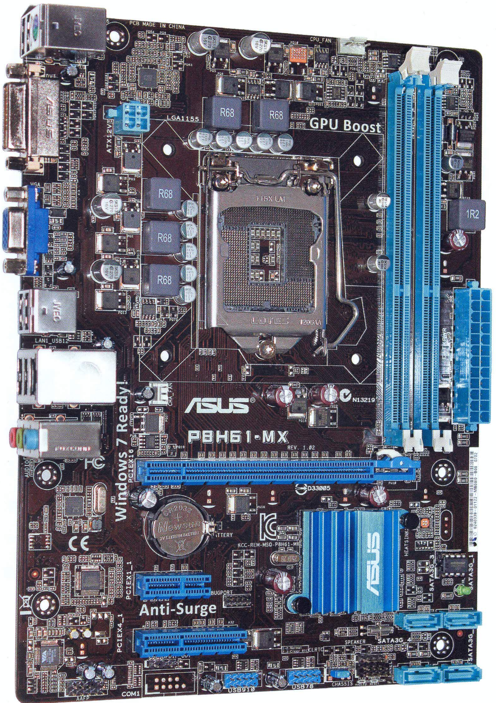
Pląta główna nr 8 (Intel, gniazdo LGA 1155)
