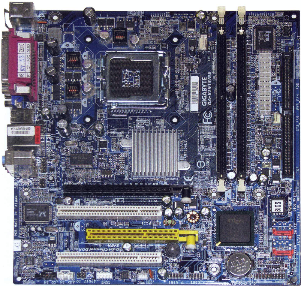
Plata główna nr 2 (Intel, gniazdo LGA 775)
