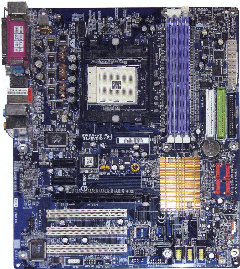
Plata główna nr 3 (AMD, gniazdo Socket 754)
